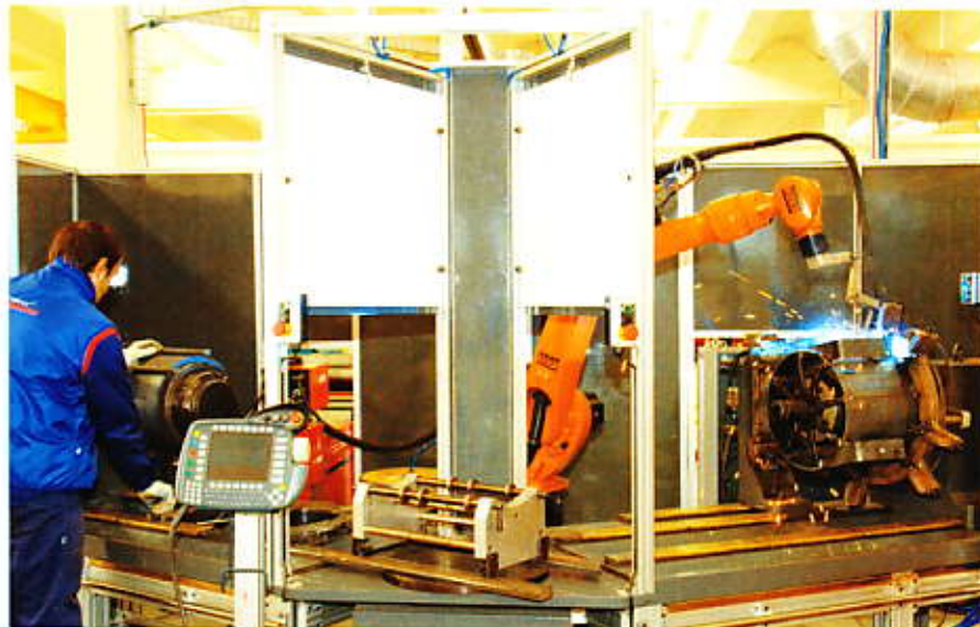
Armado y soldadura núcleos magnéticos - Assembly and welding of magnetic core.
