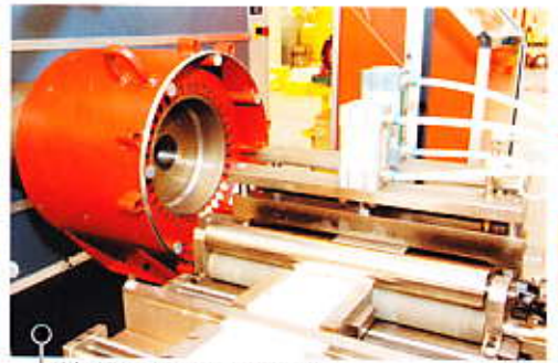
Aislación automática de ranuras Automatic slot insulation
